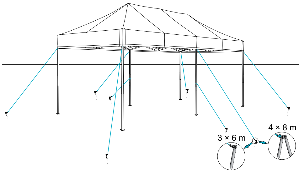
1 pav. Atramų lynų palapinėje Octa Optima II 3x6 m ir Octa Pro 3x6 m, 4x8 m montavimas
